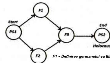
Algoritmul Holocaustului
